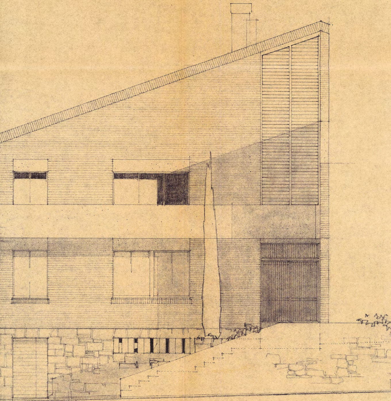
-FACHADA OESTE
